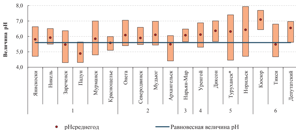
Рис. 4.42. Диапазон изменений значений pH суммарных ежемесячных проб осадков на арктических станциях в 2021 г.
