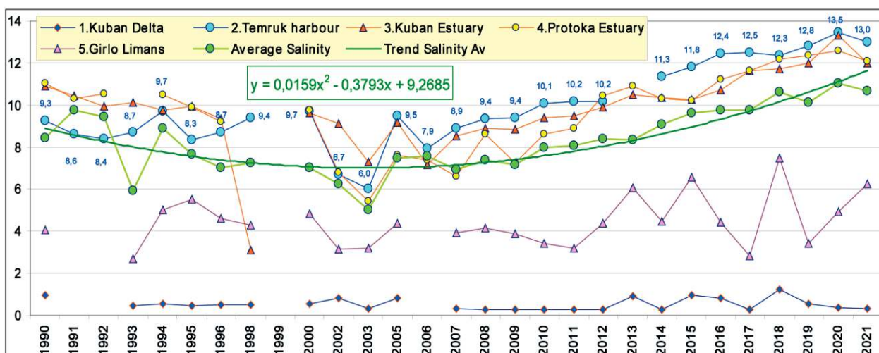
Рис. 3.59. Динамика среднегодовой солёности (%) в различных районах устьевой области р. Кубань и Темрюкском заливе в 1990-2021 гг.
