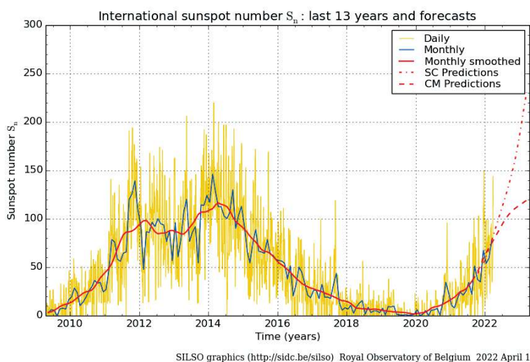
Рис. 1.1. График изменения среднемесячных значений чисел Вольфа
