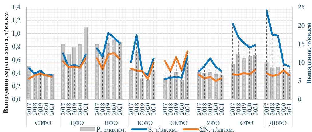
Рис. 2.20. Временной ход средних за год выпадений с осадками серы (S), суммарного азота ( \Sigma N ) и общей суммы ионов (P) по федеральным округам, 2017-2021 гг.
