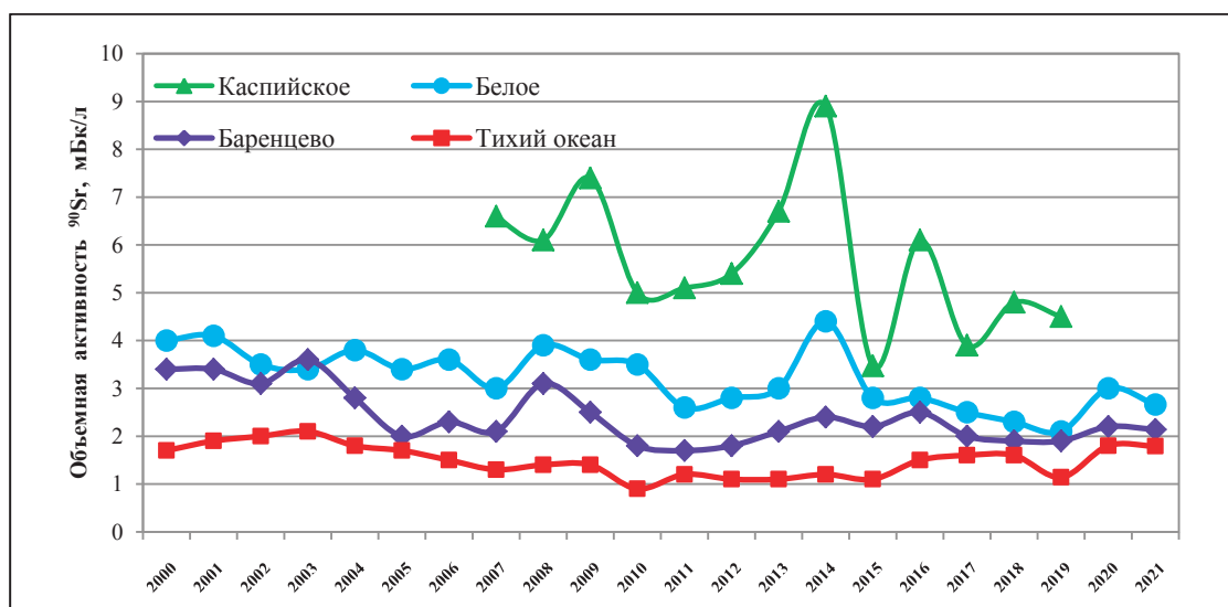
Рис. 4.60. Динамика объемной активности ^{90}\text{Sr} в прибрежных водах Белого и Баренцева морей в сравнении с водами Каспийского моря и Тихого океана вблизи восточного побережья Камчатки в 2000-2021 гг., мБк/л
