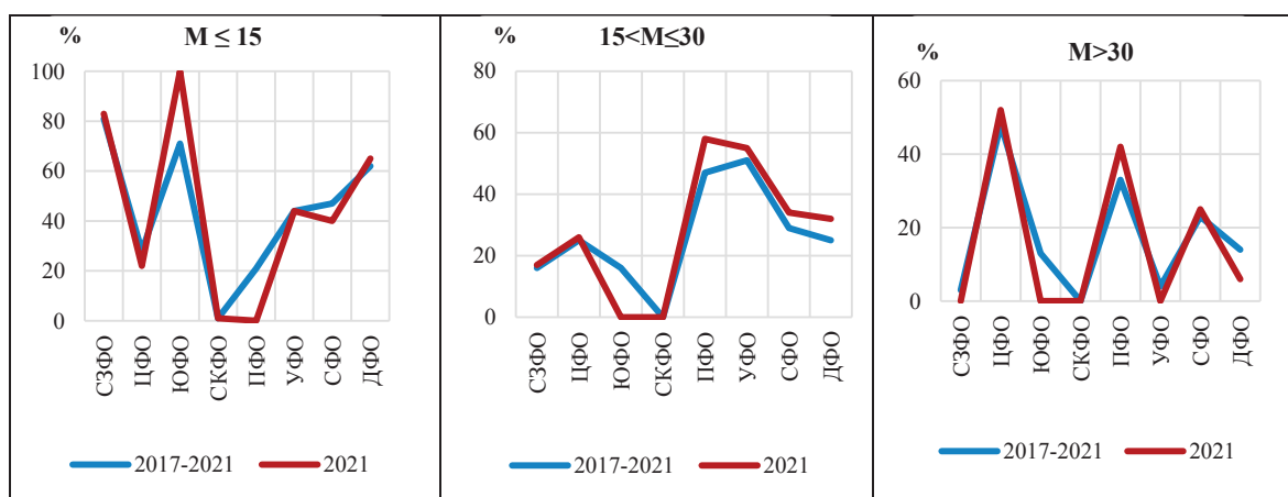
Рис. 2.19. Повторяемость (%) минерализации осадков (М) по диапазонам в период с 2017 по 2021 гг. и в 2021 г.
