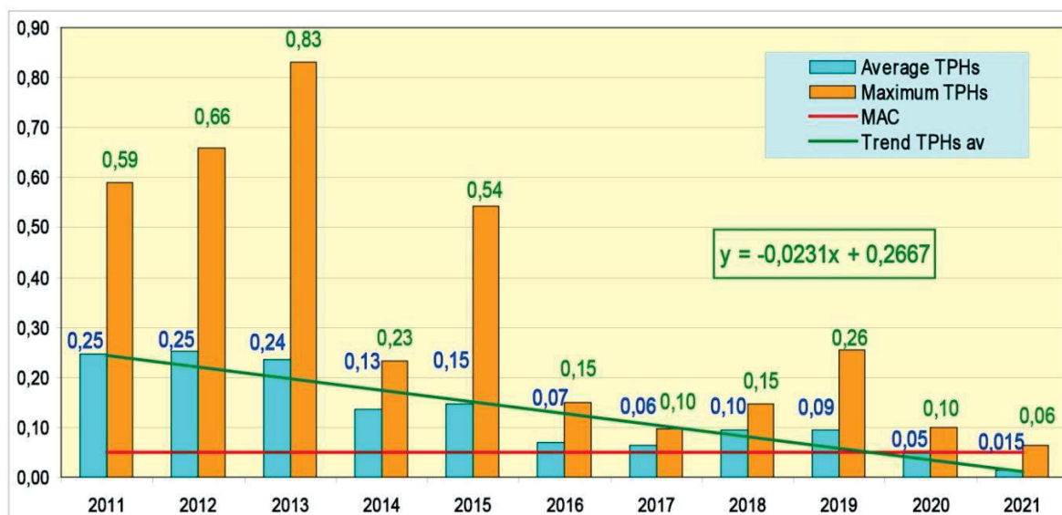
Рис. 3.67. Динамика среднегодового и максимального содержания нефтяных углеводородов (мг/дм³) в торговом порту Мурманска в 2011-2021 гг. Красная линия - ПДК (МАС).
