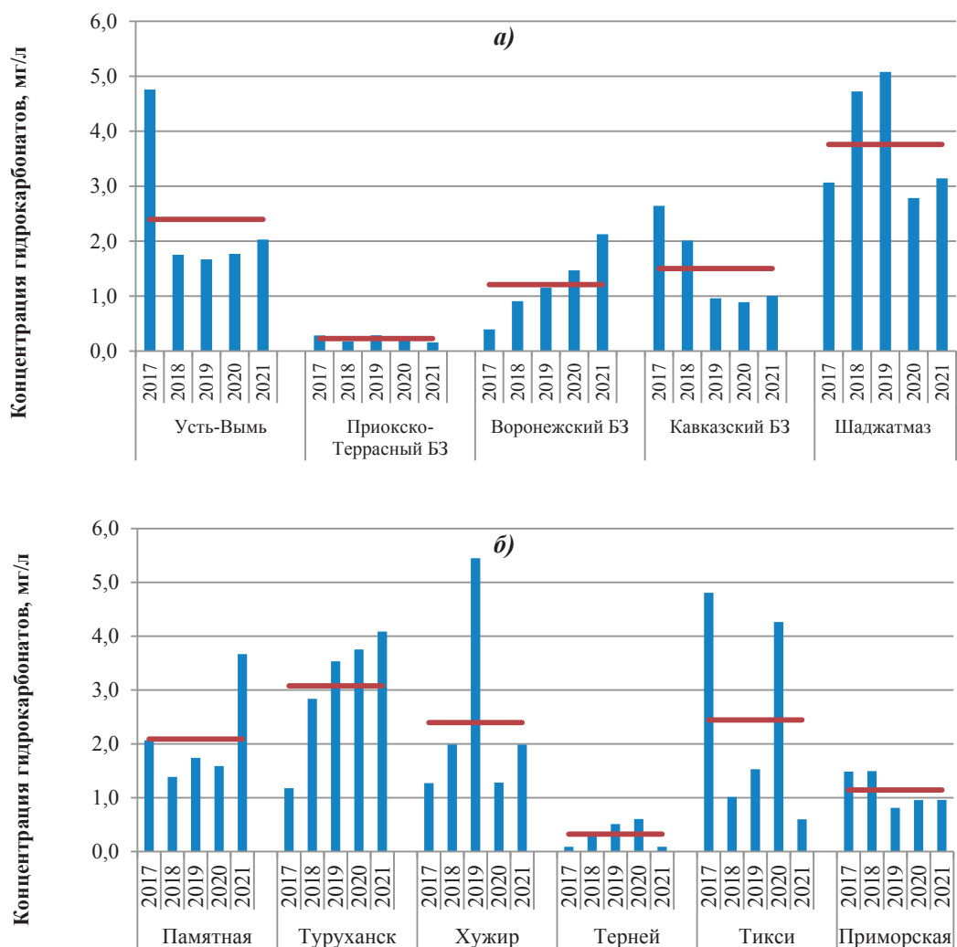
Рис. 2.16. Изменение концентрации гидрокарбонатов в осадках фоновых станций ЕЧР (а) и АЧР (б), 2017-2021 гг.
