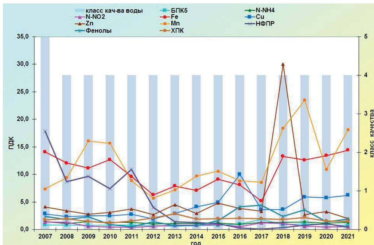
Рис. 3.43. Изменение среднегодовых концентраций отдельных загрязняющих веществ и показателей качества воды р. Обь ниже г. Салехард за многолетний период
