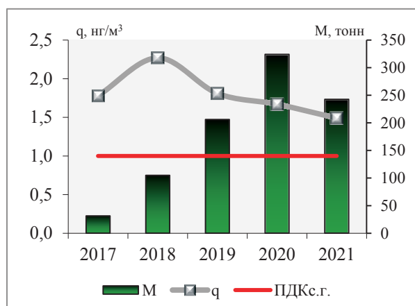
Рис. 3.13. Среднегодовые концентрации бенз(а)пирена ( q , нг/м 3 ) и выбросы от стационарных источников ( M , тонн)
