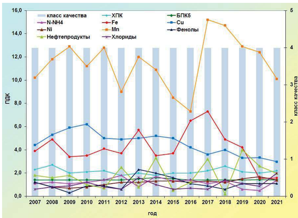
Рис 3.40. Изменение среднегодовых концентраций отдельных загрязняющих веществ и показателей качества воды р. Белая, 10,5 км ниже г. Sterлитамак
