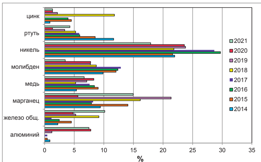
Рис. 4.49. Распределение числа случаев ВЗ и ЭВЗ по ингредиентам (в % от общего количества случаев ВЗ и ЭВЗ Арктической зоны РФ)
