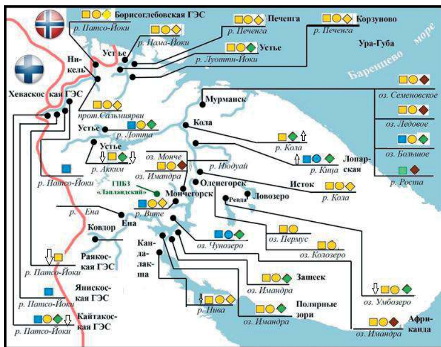
Рис. 4.55. Картограмма качества вод Мурманской области по гидробиологическим показателям в 2021 г.
