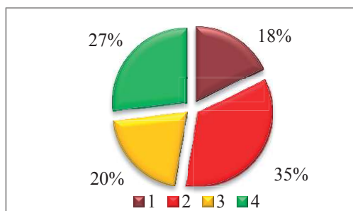
Рис. 3.15. Количество городов (%), где ИЗА \geq 14 (1), 7-13 (2), 5-6 (3), \leq 5 (4)
