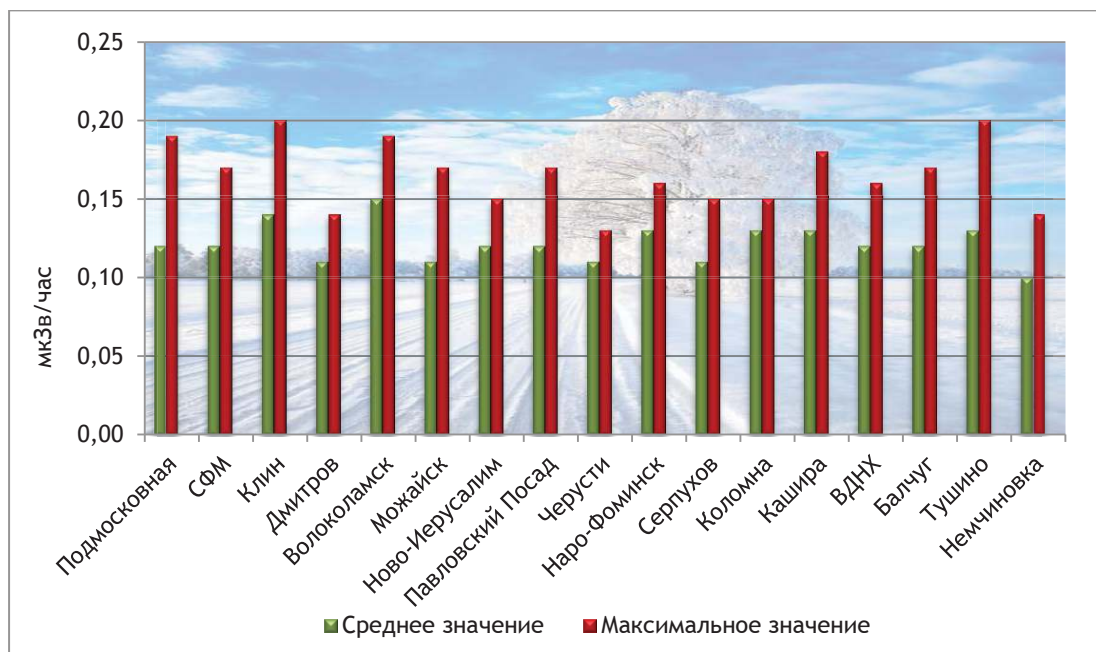
Рис. 4.8. Мощность амбиентного эквивалента дозы гамма-излучения (МАЗД) на станциях Московского региона в 2021 г.
