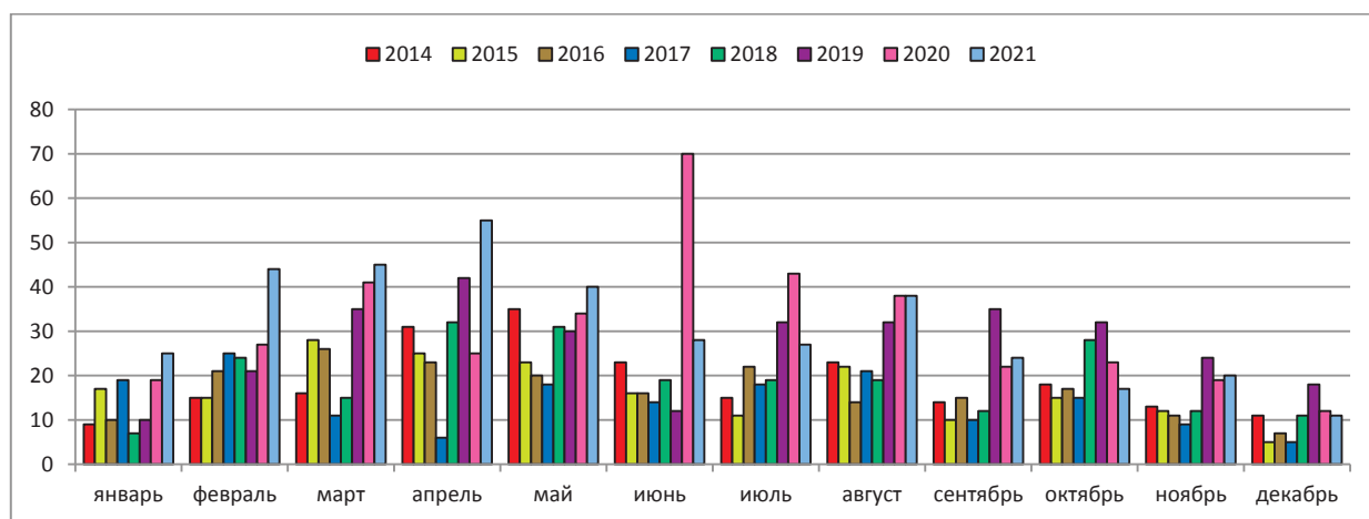
Рис. 4.50. Динамика внутригодичного распределения случаев ВЗ и ЭВЗ поверхностных вод Арктической зоны РФ за период 2014-2021 гг.
