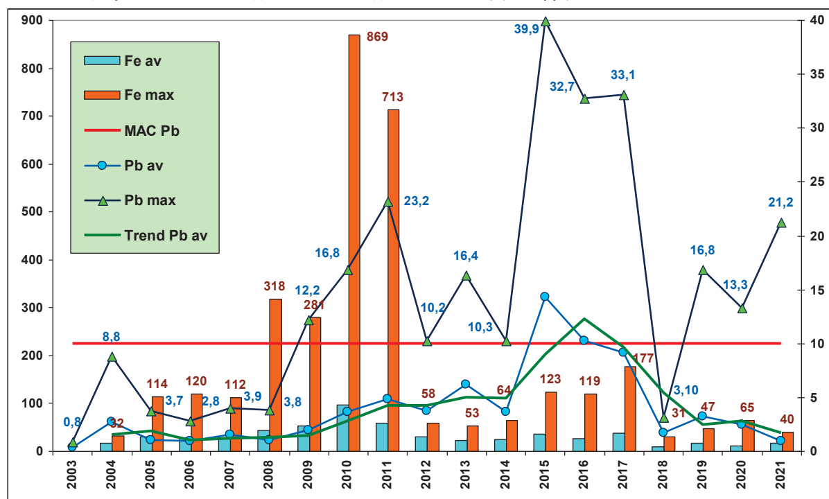
Рис. 3.64. Средняя и максимальная концентрации железа и свинца (мкг/дм³) в прибрежных водах района Адлер-Сочи в 2003-2021 гг.
