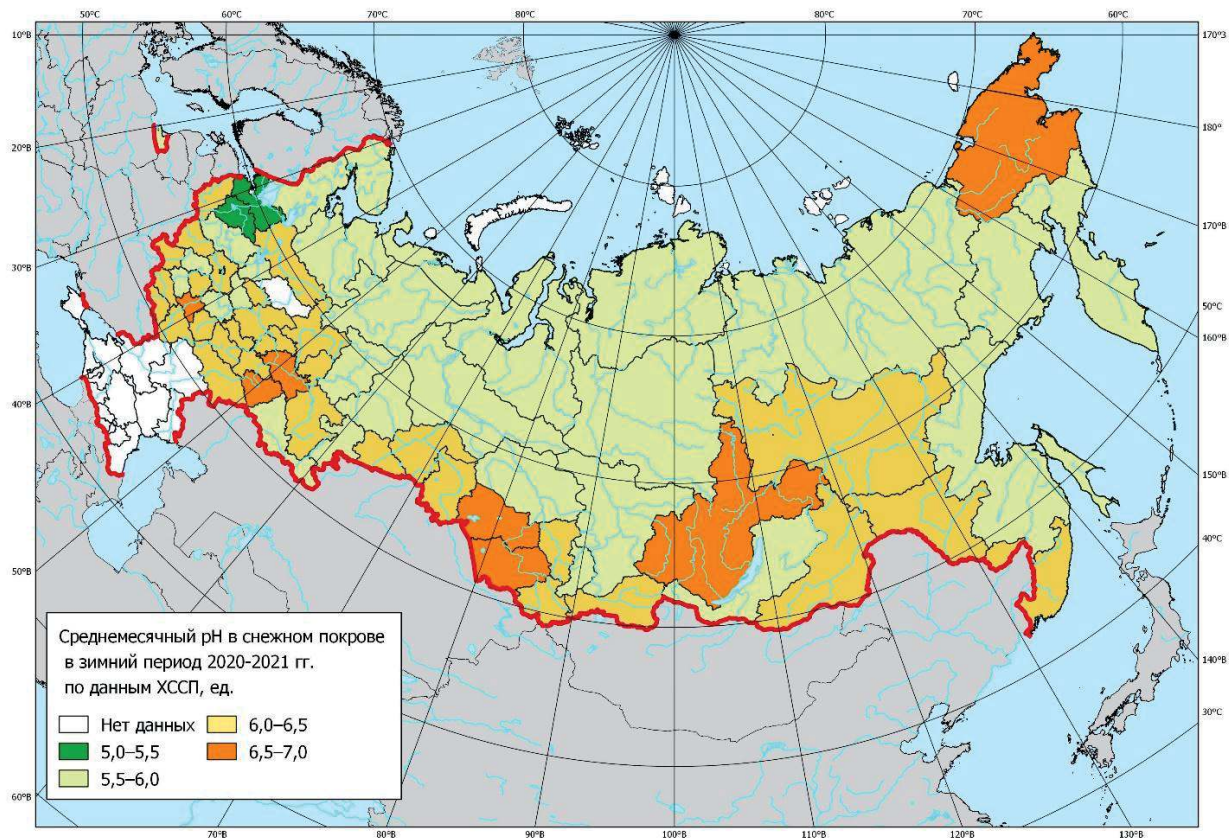
Рис. 2.23. pH снежного покрова в зимний период 2020-2021 гг.
