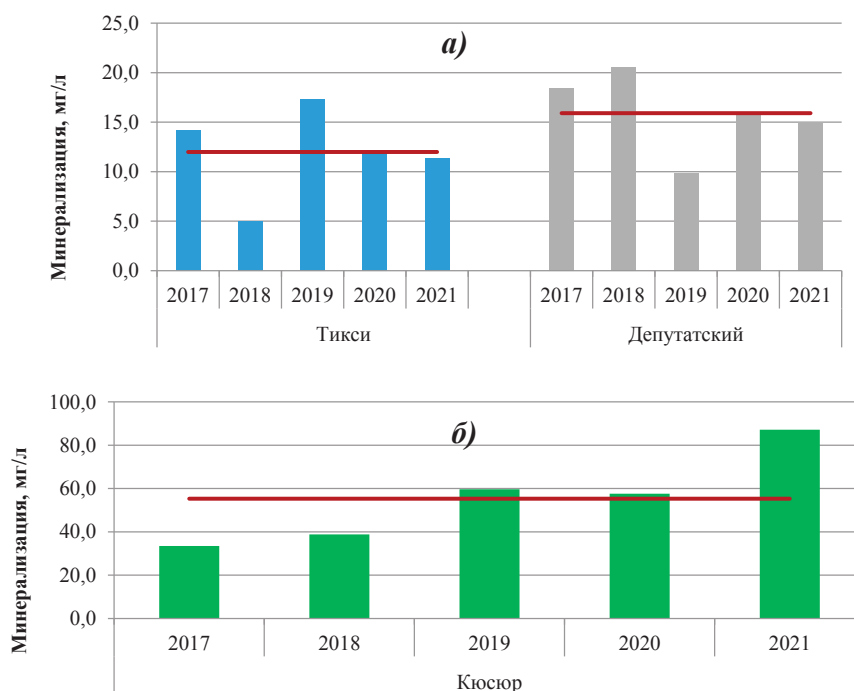
Рис. 4.41. Изменение средневзвешенной минерализации осадков на территории Якутии, 2017-2021 гг.
