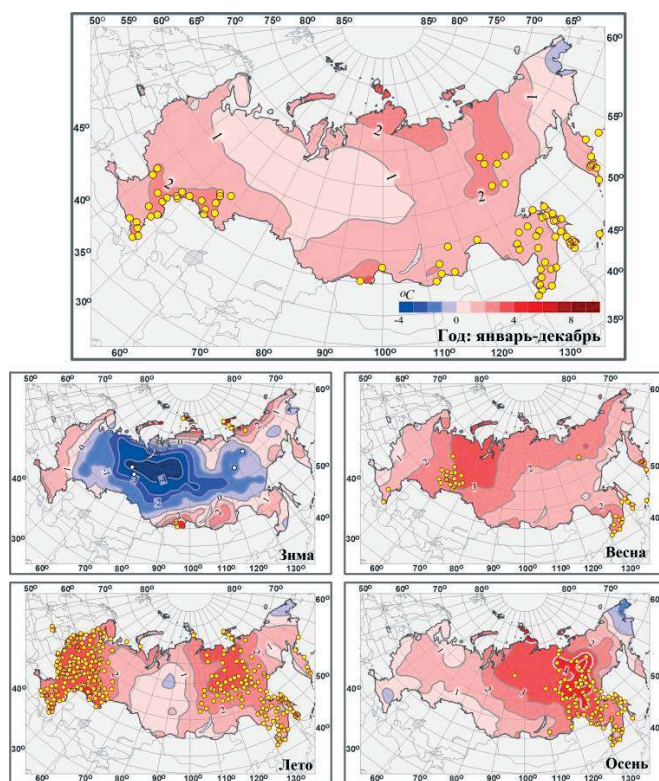
Рис. 1.8. Аномалии средней годовой и сезонных температур приземного воздуха на территории России в 2021 г. (отклонения от средних за 1961-1990 гг.) с указанием локализации экстремальных аномалий.
