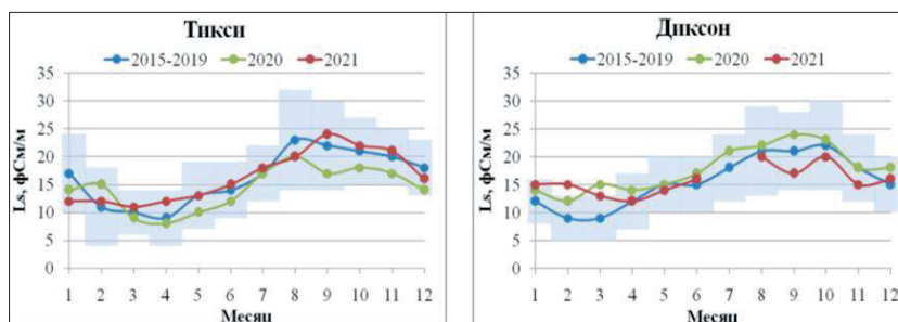
Рис. 4.35. Годовой ход L s на станциях Тикси и Диксон за 2021 г. в сравнении с 2020 г. и на фоне осредненного годового хода L s за предшествующий период
