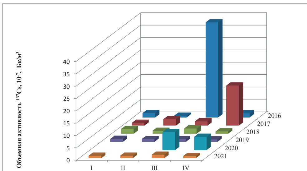
Рис. 4.59. Динамика средней за квартал величины объемной активности ^{137}\text{Cs} в воздухе в Мурманске в 2016-2021 гг.
