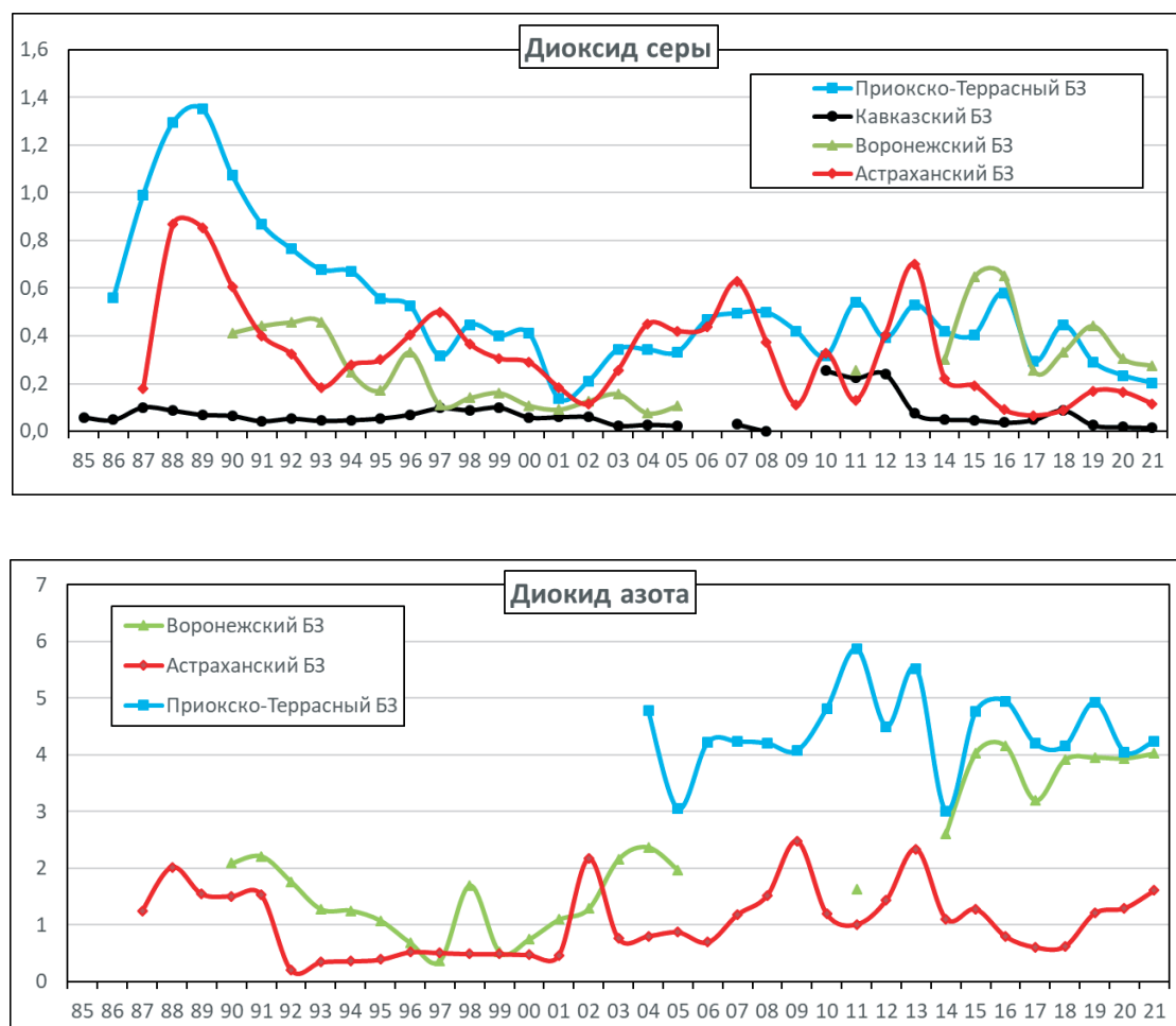
Рис. 2.14. Изменение фоновое содержания диоксида серы и диоксида азота в атмосферном воздухе фоновых районов (мкг/м³)
