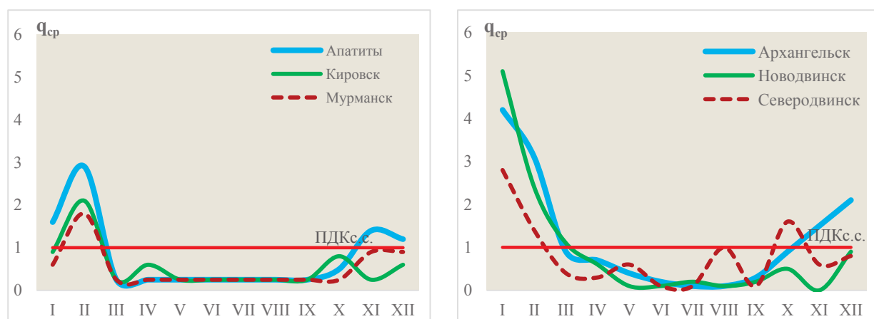
Рис. 4.47. Годовой ход бенз(а)пирена в городах АЗРФ в 2021 г., q_{cp} , ng/m^3
