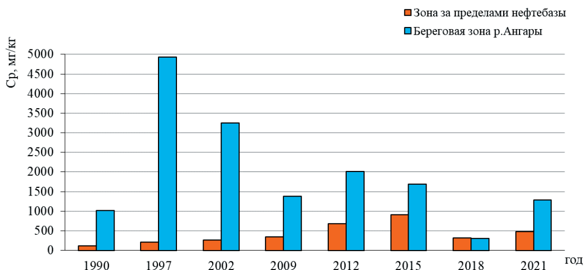
Рис. 3.27. Динамика изменения содержания нефтепродуктов в почвах за пределами Жилкинской нефтебазы г. Иркутска и береговой зоны р. Ангары
