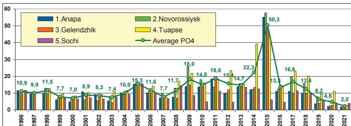
Рис. 3.63. Динамика средней концентрации фосфатов P-PO 4 (мг/дм³) в прибрежных водах Кавказа в 1996-2021 гг.
