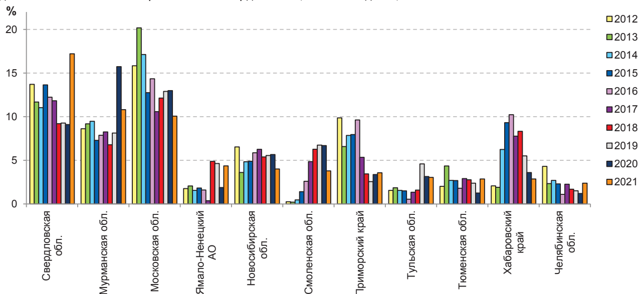
Рис. 3.51. Динамика количества случаев ВЗ и ЭВЗ по субъектам Российской Федерации, в которых регистрировалось наибольшее количество случаев ВЗ и ЭВЗ в 2021 г. (в % от общего количества случаев ВЗ и ЭВЗ на территории Российской Федерации)
