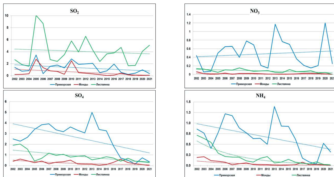
Рис. 2.28. Изменения средних годовых концентрации соединений серы (слева) и азота (справа) в воздухе на станциях ЕАНЕТ (мкг/м 3 )
