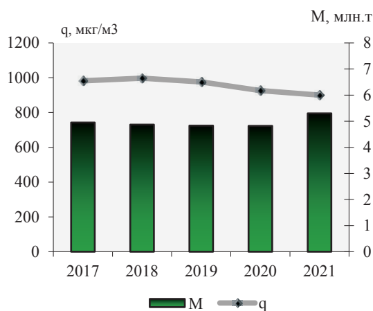
Рис. 3.11. Среднегодовые концентрации ( q , мкг/м 3 ) и выбросы от стационарных источников ( M , млн. т) оксида углерода
