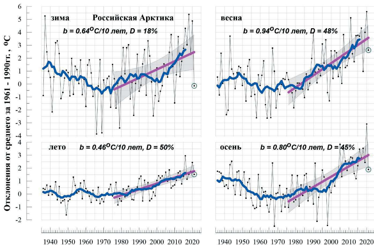
Рис. 4.27. Сезонные аномалии температуры воздуха в Российской Арктике в 1936-2021 гг. Жирная синяя кривая - 11-летнее скользящее среднее. Показан линейный тренд за 1976-2021 гг.
