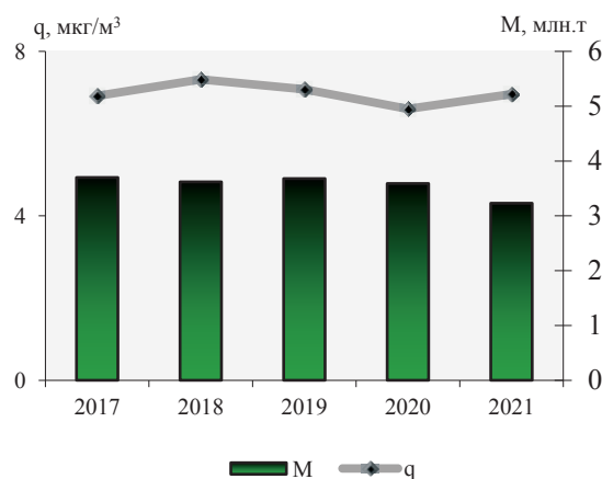
Рис. 3.10. Среднегодовые концентрации ( q , мкг/м 3 ) и выбросы от стационарных источников ( M , млн. т) диоксида серы
