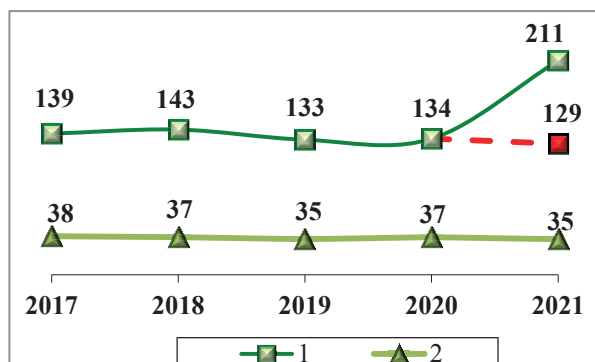
Рис. 3.3. Количество городов, в которых среднегодовые концентрации одного или нескольких веществ превышали 1 ПДК с учетом прежних (2017-2021 гг.) и новых (2021 г.) нормативов (1), и отмечались значения СИ больше 10 (2)
