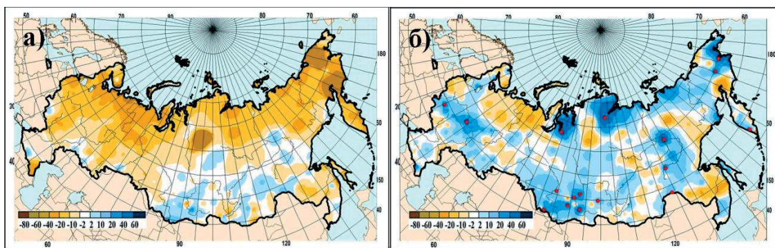
Рис. 1.13. а) Аномалии числа дней с покрытием снегом более 50% территории вокруг метеорологических станций зимой 2020-2021 гг. (от среднемноголетних значений за период 1971-2000 гг.);
