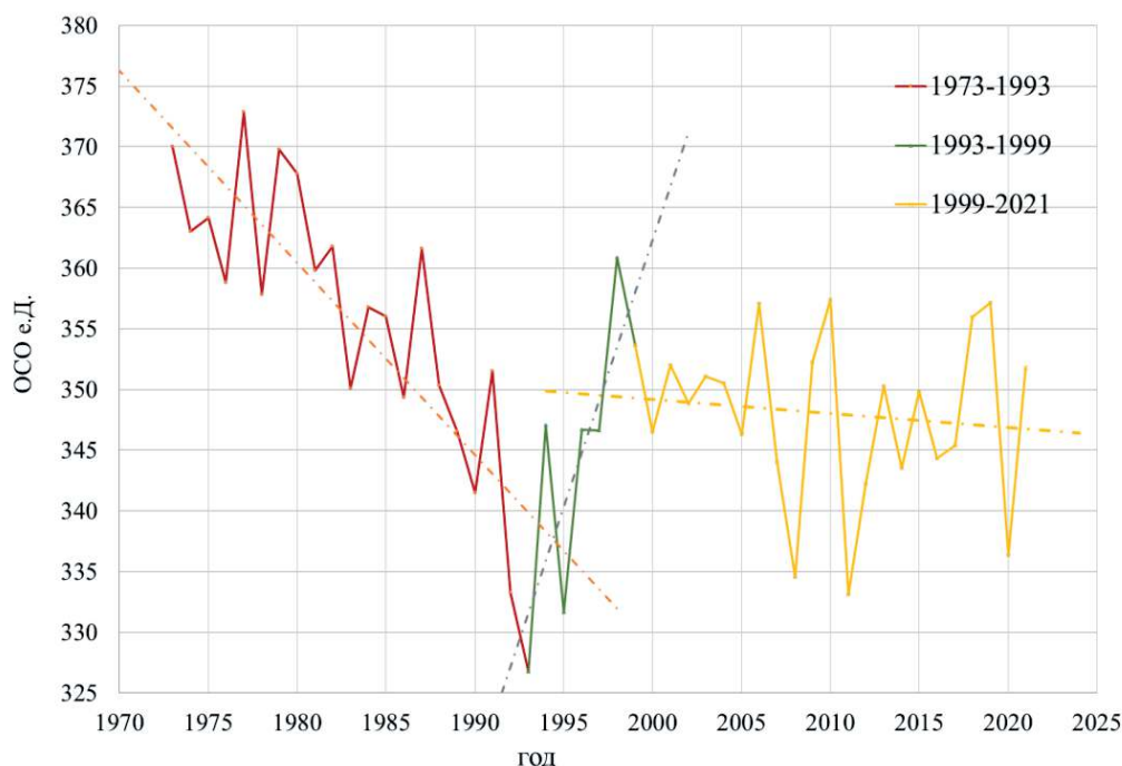
Рис. 2.11. Среднегодовые значения ОЗО над территорией РФ в период 1973-2021 гг.
