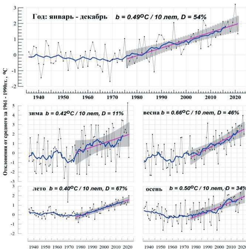
Рис. 1.7. Средние годовые (вверху) и сезонные аномалии температуры приземного воздуха ( ^{\circ}\text{C} ), осредненные по территории РФ, 1936-2021 гг.
