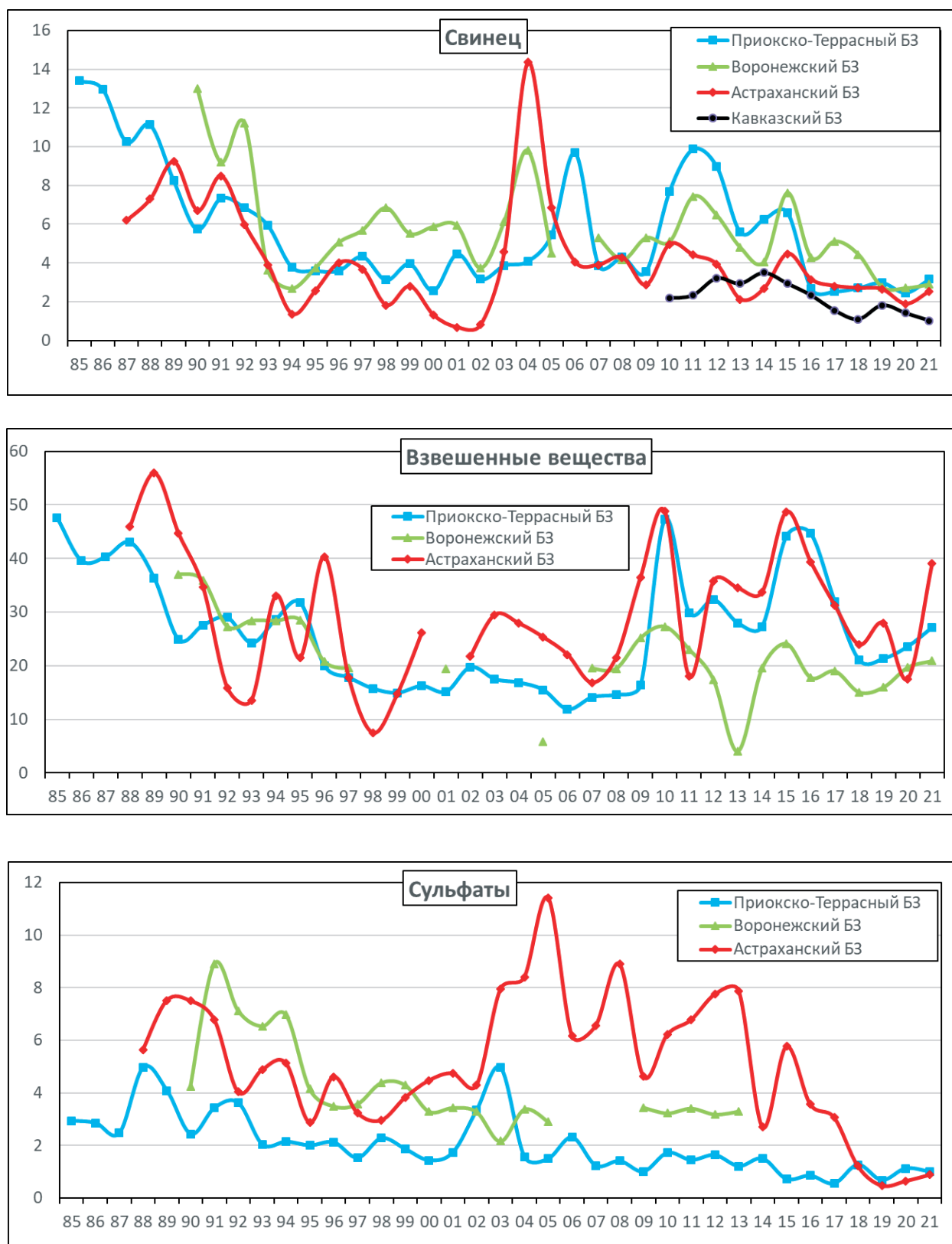
Рис. 2.13. Изменение среднегодового содержания свинца ( \text{нг/м}^3 ), взвешенных веществ и сульфатов ( \text{мкг/м}^3 ) в атмосферном воздухе фоновых районов
