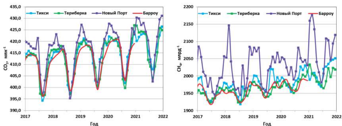
Рис. 2.1. Временной ход концентраций CO 2 и CH 4 на российских арктических станциях в сравнении с данными станции Барроу (НУОА, США)
