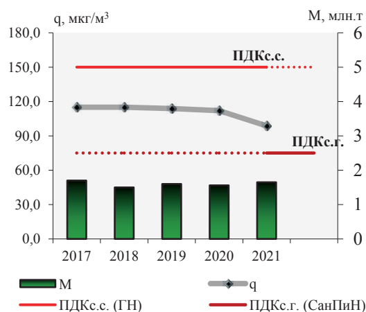
Рис. 3.9. Среднегодовые концентрации ( q , мкг/м 3 ) взвешенных веществ и выбросы от стационарных источников ( M , млн. т) твердых веществ
