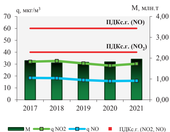
Рис. 3.12. Среднегодовые концентрации диоксида ( qNO_2 , мкг/м 3 ) и оксида азота ( qNO , мкг/м 3 ) и выбросы от стационарных источников ( M , млн. т) NO_x (в пересчете на NO_2 )
